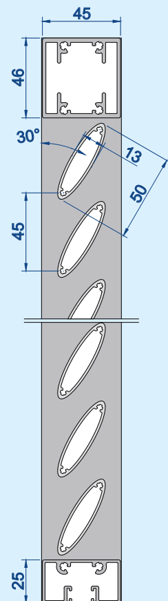
Vertikalschnitt: Maßstab 1:3
